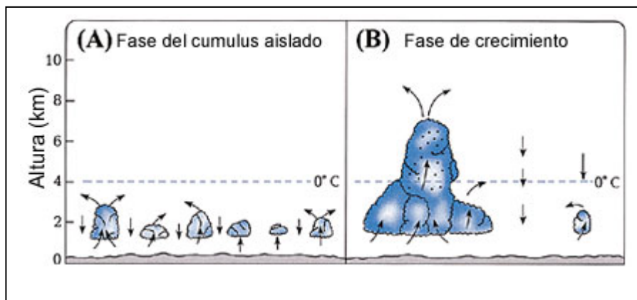
Figura 19: (A) Pequeños pedazos sueltos de nubes (cúmulos). (B) Cuando las pequeñas nubes se juntan las corrientes de aire en la gran nube aumentan, haciendo que la nube vaya tomando la forma de una pila. Las gotas de agua están indicadas con (.). ( The Atmosphere [La Atmósfera], Anthes y otros, p. 269.)
