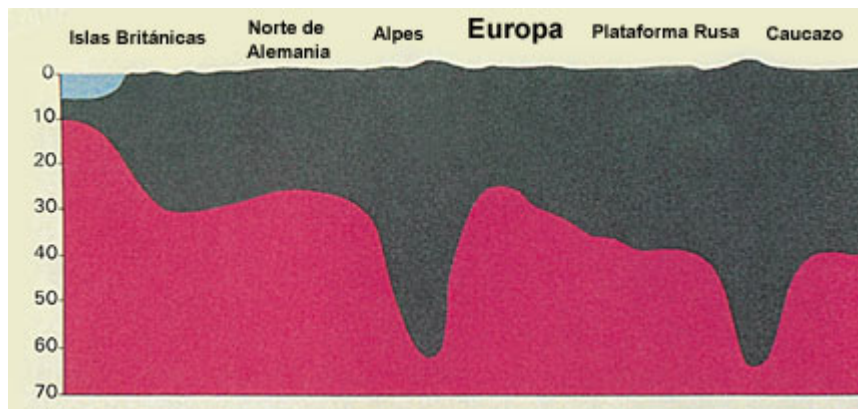
Figura 8: Corte esquemático. Las montañas, al igual que las estacas, tienen raíces profundas, enterradas en el suelo. ( Anatomy of the Earth [Anatomía de la Tierra], Cailleux, p. 220.)
