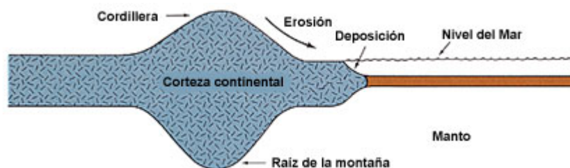
Figura 9: Otra ilustración muestra como las montañas tienen forma de "estaca", debido a sus profundas raíces. ( Earth Science [Ciencia de la Tierra], Tarbuck y Lutgens, p. 158.)
