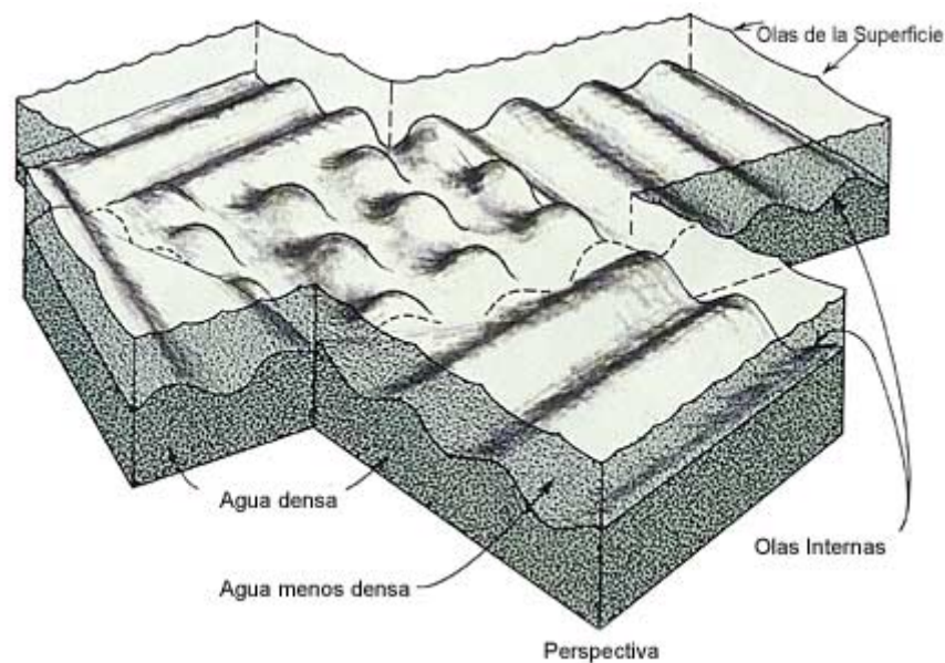
Figura 16: Olas internas en la zona intermedia entre dos estratos de agua con diferentes densidades. Una es densa (la de más abajo), y la otra es menos densa (la de más arriba). ( Oceanography ) Oceanografía , Gross, p. 204.)
