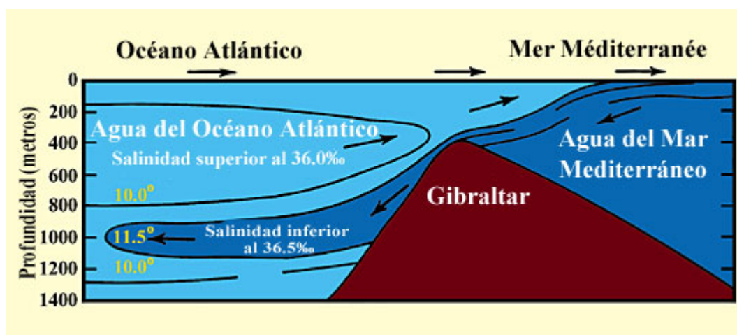
Figura 13: El agua del Mediterráneo al entrar en el Atlántico por encima del estrecho de Gibraltar todavía con su propia temperatura, salinidad y menor densidad, debido a la barrera que distingue entre ellas. Las temperaturas están en grados Centígrados (C°) (Levemente modificado de The Marine Geology [La Geología Marina], Kuenen, p. 43.)
