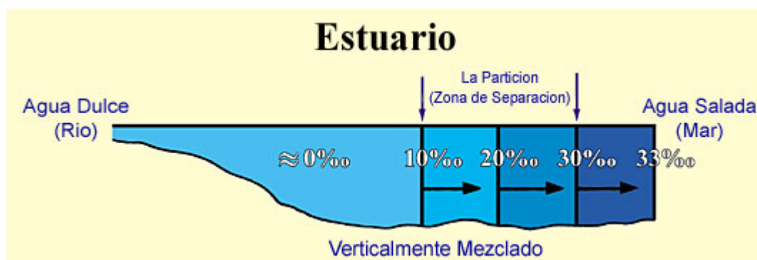
Figura 14: Corte longitudinal que muestra la salinidad (partes por mil 0/00), en un estuario. Aquí podemos observar la partición (Zona de separación), entre el agua dulce y la salada. (Levemente modificado de Introductory Oceanography [Oceanografía Introductoria], Thurman, p. 301.)
