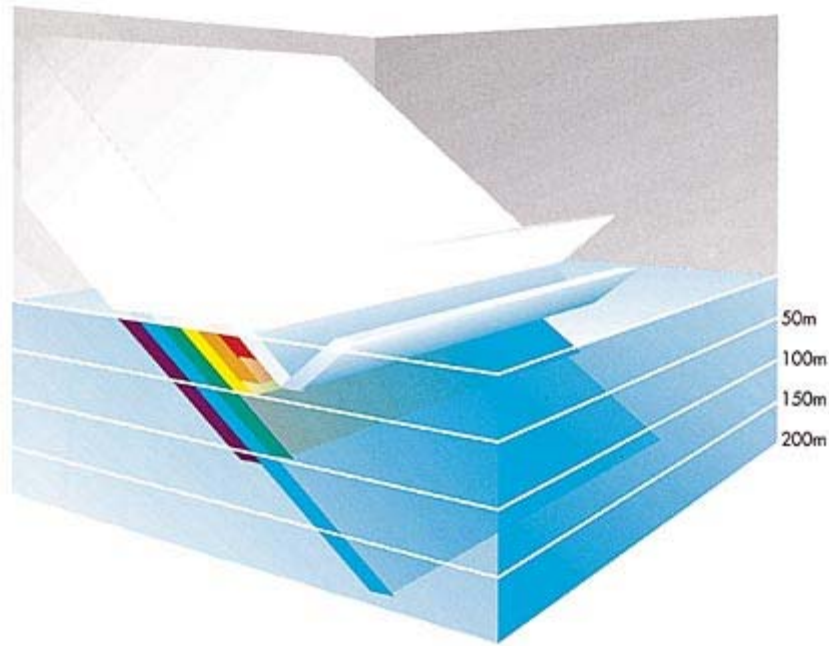
Figura 15: Entre el 3 y el 30% de la luz solar es reflejada en la superficie marina. Luego, casi todos los siete colores del espectro son absorbidos uno tras otro en los primeros 200 mts, excepto la luz azul. ( Oceans [Los Océanos], Elder y Pernetta, p. 27.)
